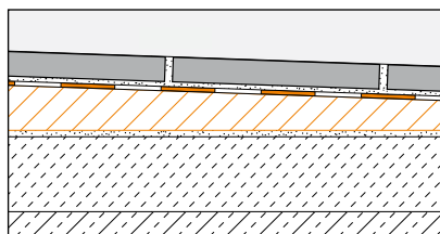
Schlüter®-KERDI-SHOWER sur chape
