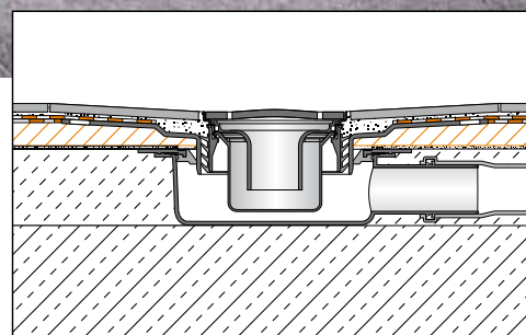
Évacuation horizontale
